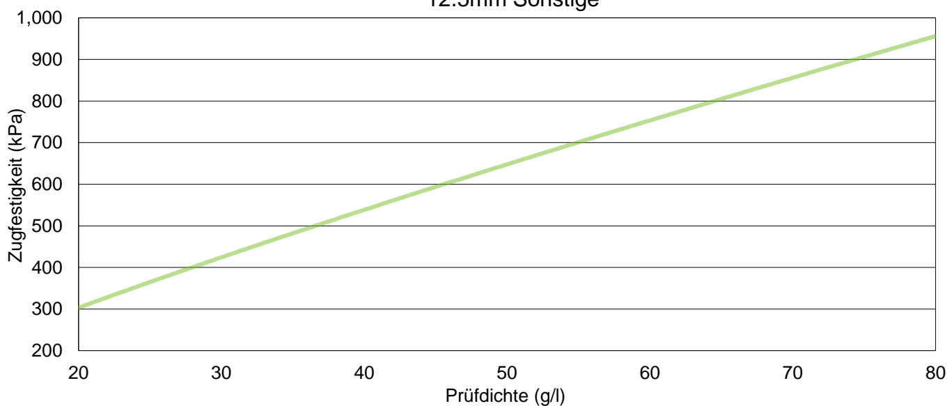
Zugfestigkeit - ISO 1798 12.5mm Sonstige
