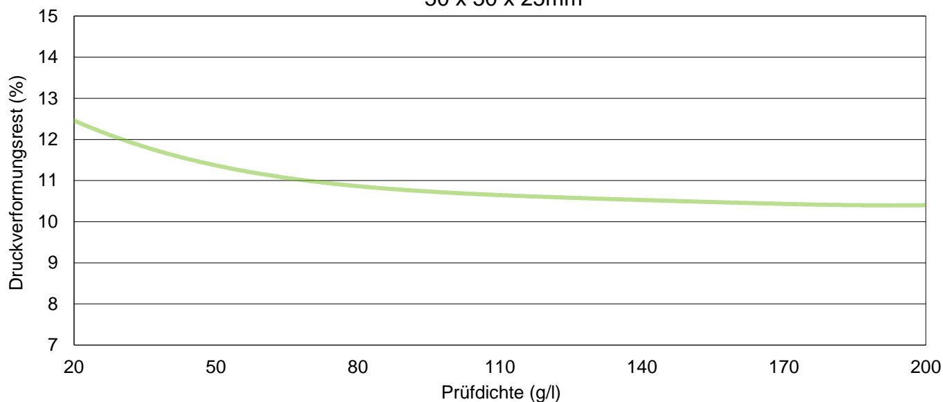
Druckverformungsrest - ISO 1856 C 50 x 50 x 25mm
