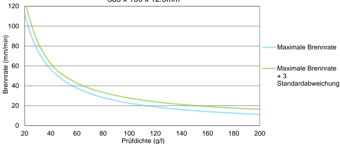
Brennrate in Abhängigkeit von der Dichte - ISO 3795 365 x 100 x 12.5mm
