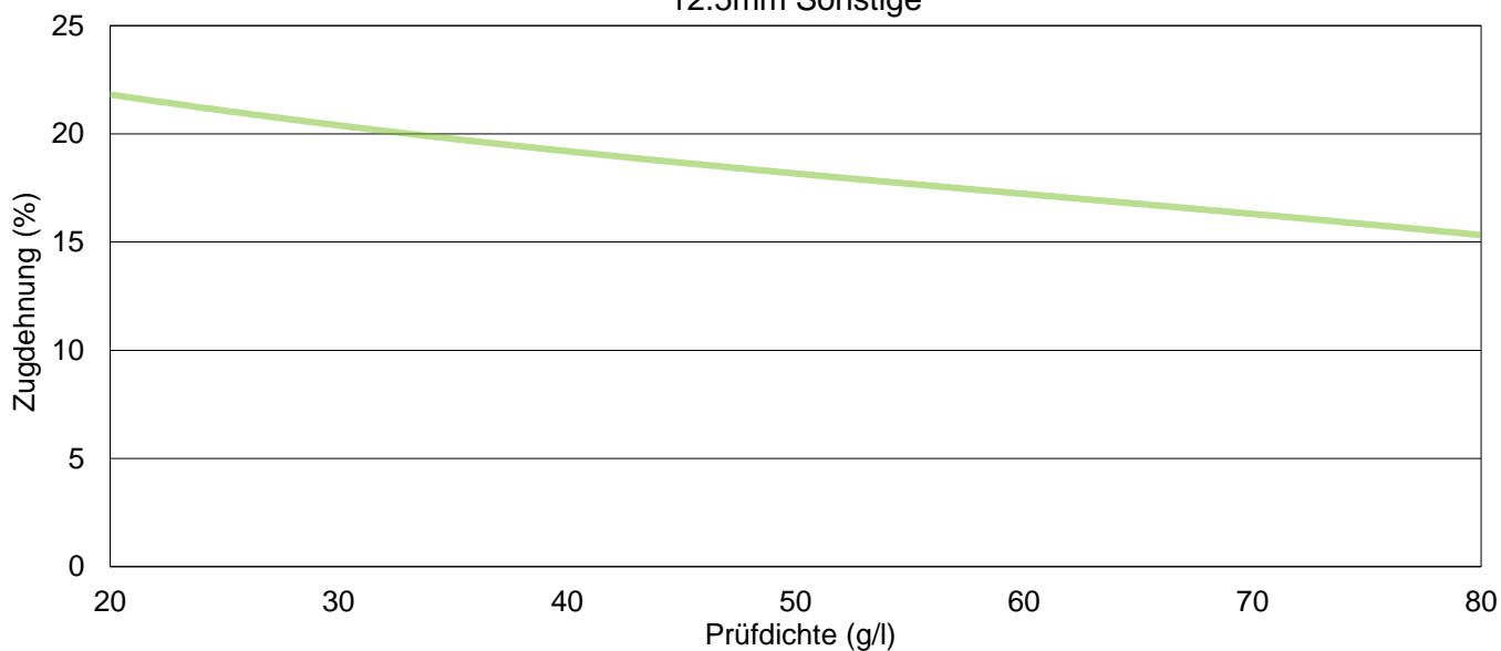
Zugdehnung - ISO 1798 12.5mm Sonstige
