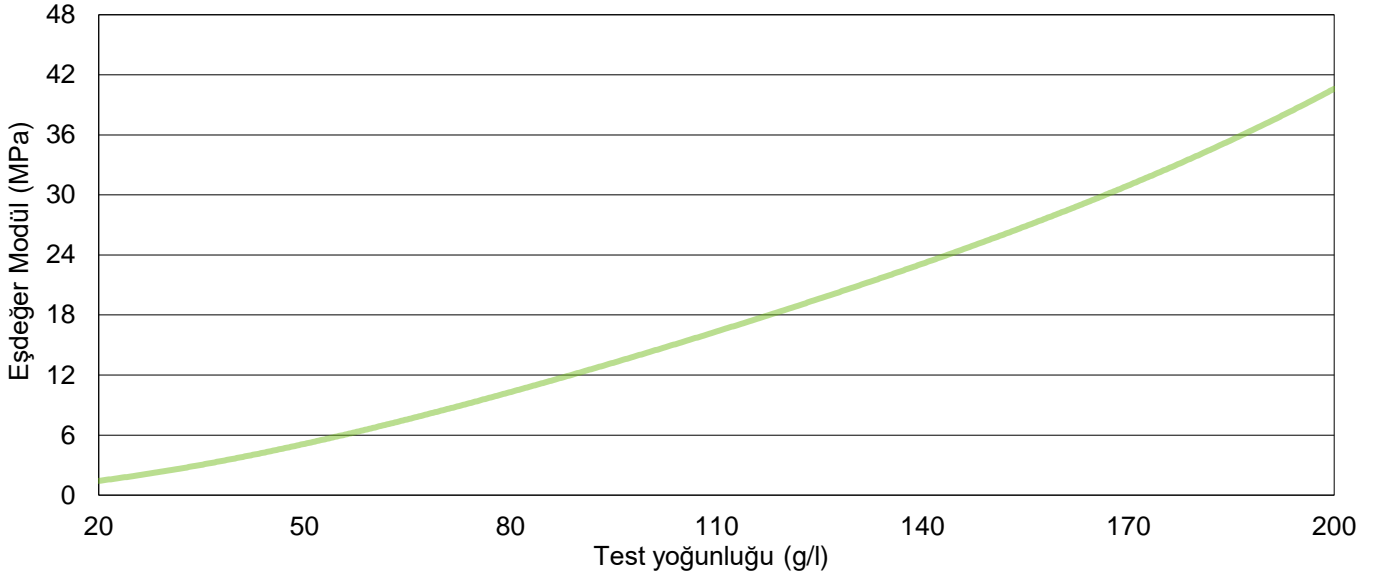
Eşdeğer Modül %3'lük sıkırtmada - ISO 844 50 x 50 x 50mm
