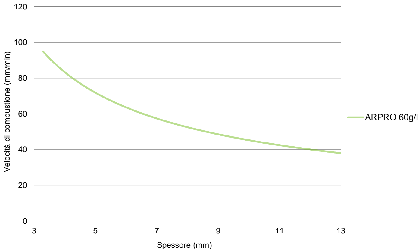
Velocità di combustione vs spessore - ISO 3795
