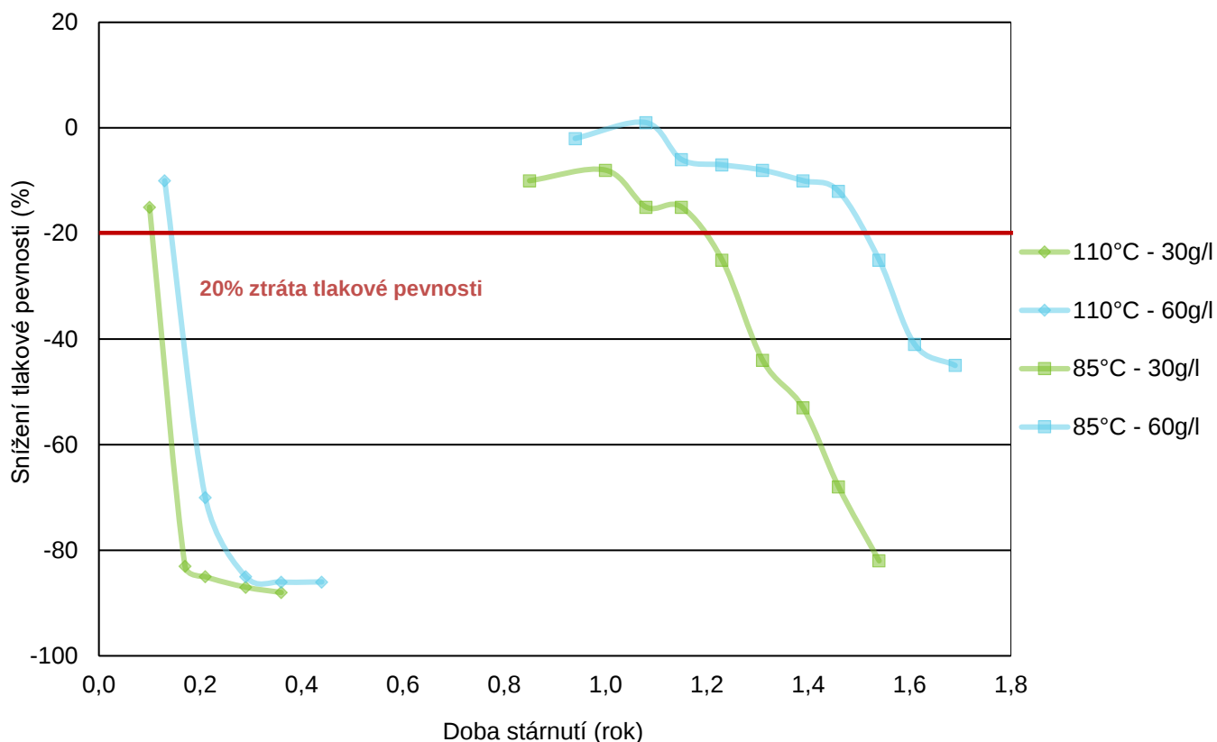
Ztráta tlakové odolnosti v důsledku stárnutí
