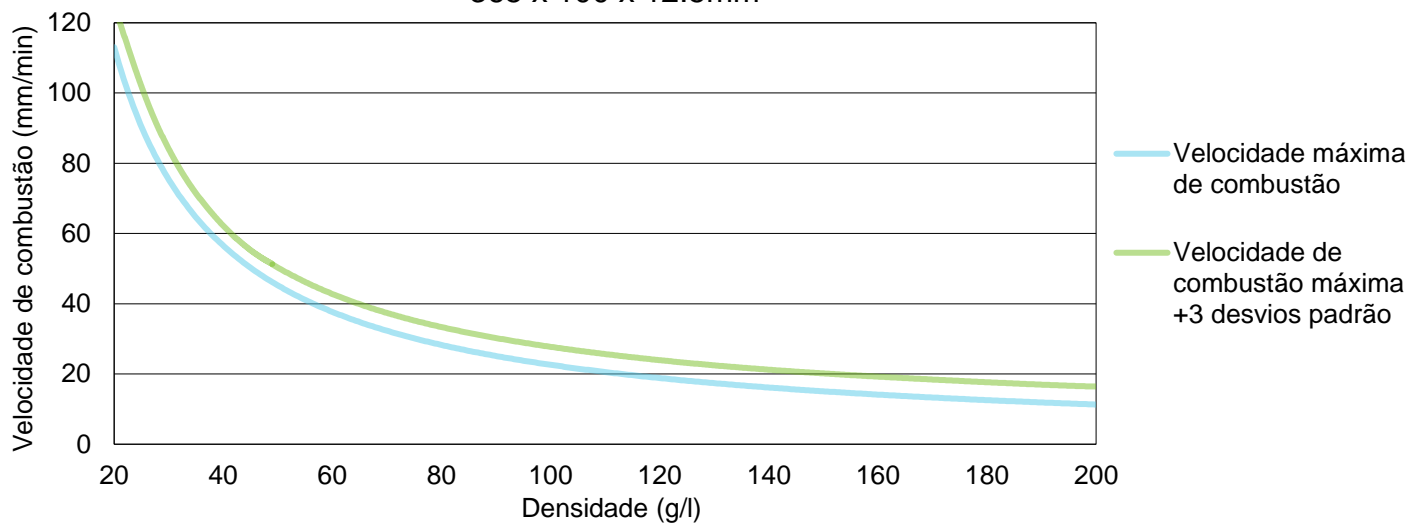
Velocidade de combustão vs densidade - ISO 3795 365 x 100 x 12.5mm
