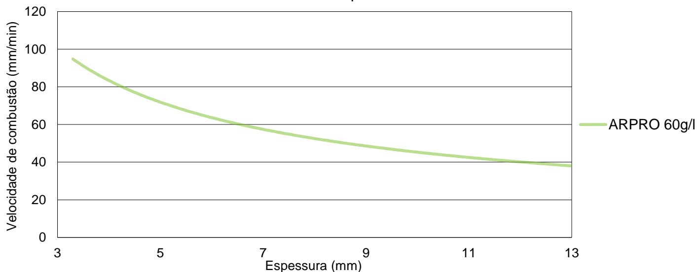
Velocidade de combustão vs espessura - ISO 3795
