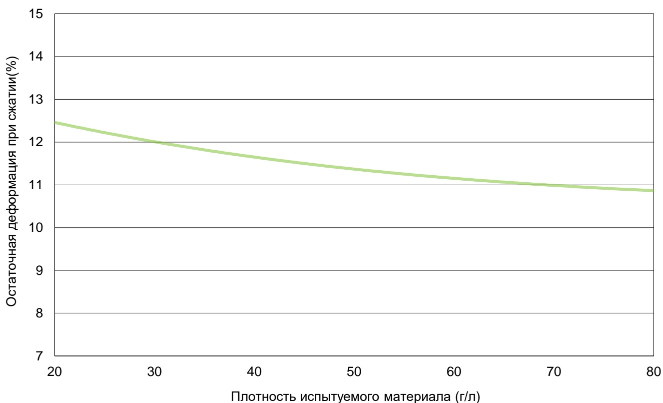
Остаточная деформация при сжатии - ISO 1856 C
