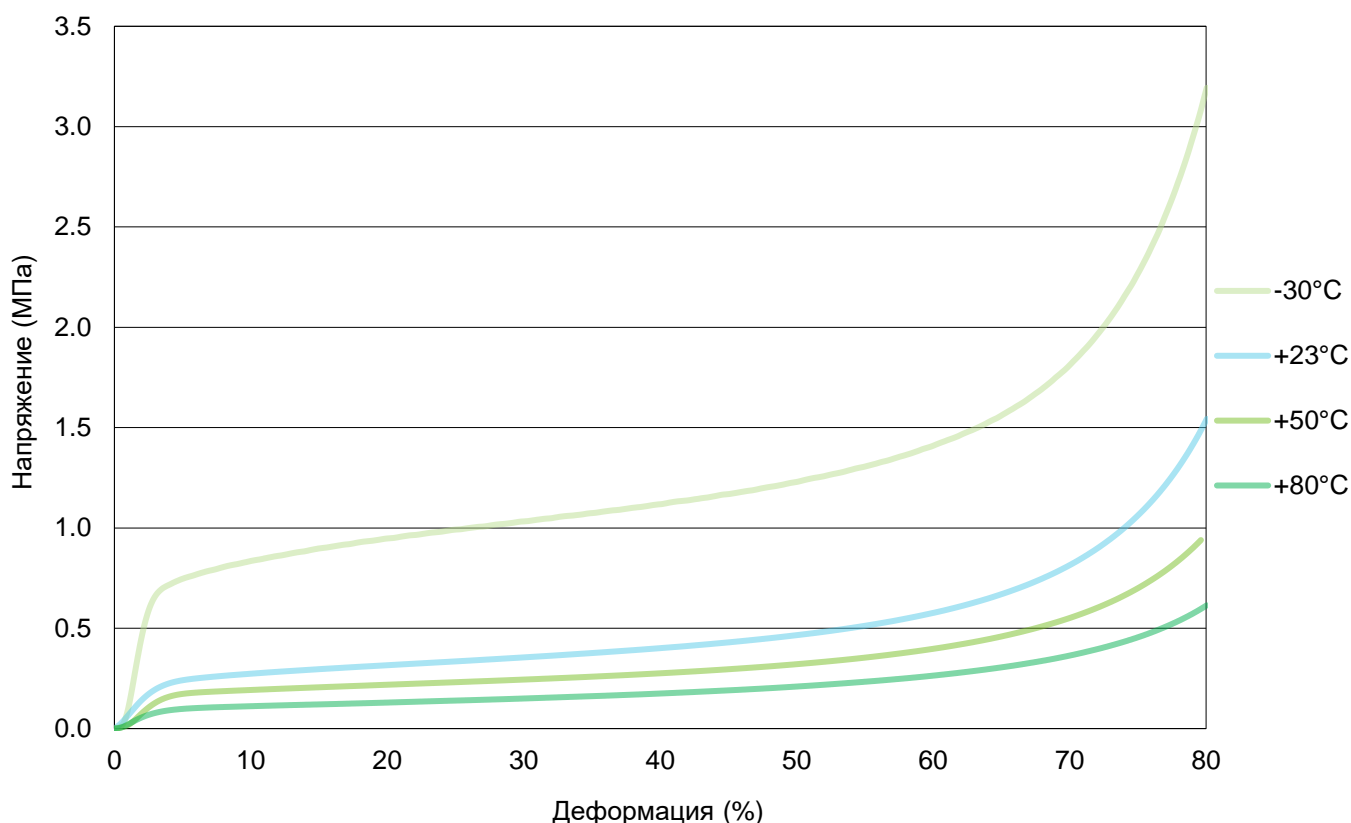
Свойства под сжимающей нагрузкой - ISO 844
