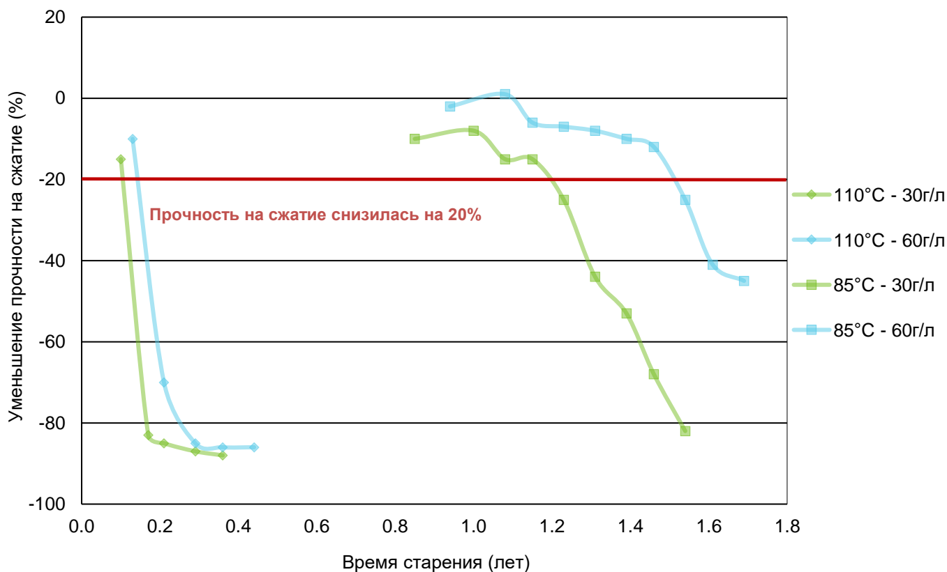
Потеря прочности на сжатие в результате старения
