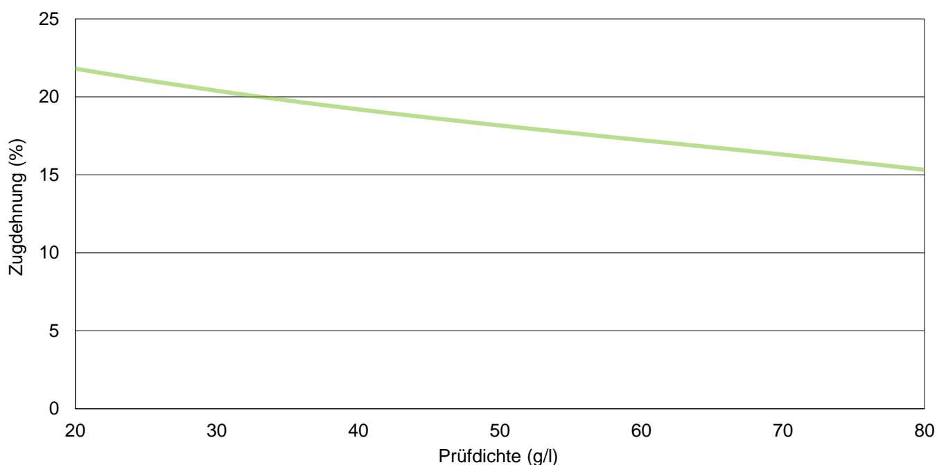
Zugdehnung - ISO 1798
