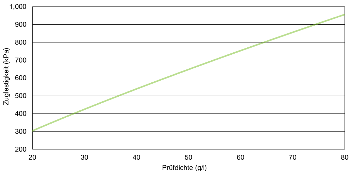
Zugfestigkeit - ISO 1798
